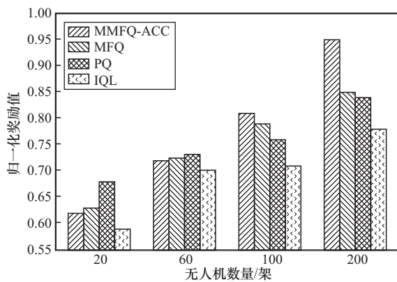
图4 无人机数量对算法性能的影响
