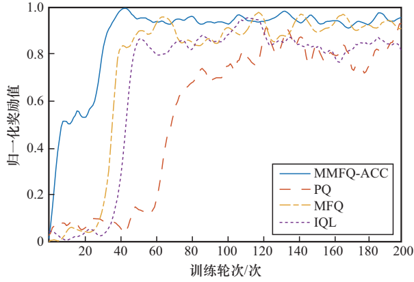
图8 不同算法收敛性比较
