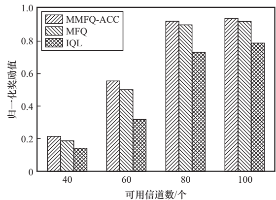
图5 不同算法的归一化奖励值随可用信道数变化的对比
