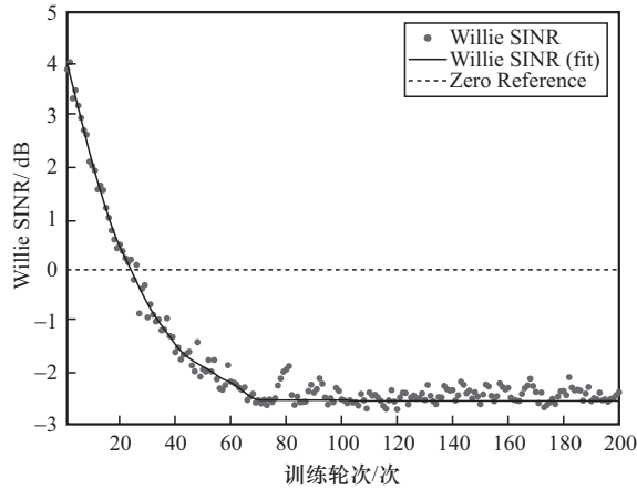
图6 MMFQ-ACC 算法下 Willie SINR 随训练轮次变化的趋势
