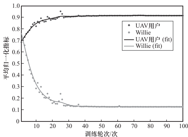
图7 UAV 用户与 Willie 平均归一化指标随训练轮次变化的对比
