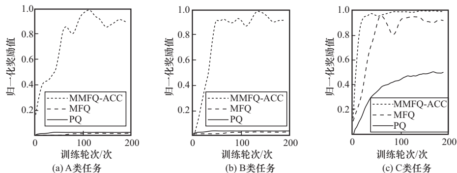
图 10 不同任务场景下归一化奖励值随训练轮次变化情况
