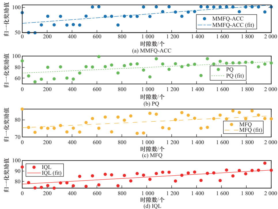
图9 归一化奖励值随时隙数变化情况
